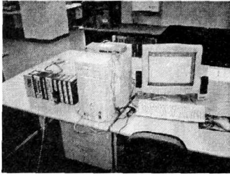
(b) 그림 1. 고막온의 측정(a)과 측정 시스템(b) Fig 1. measurement of tympanic temperature(a) & measurement system(b)
